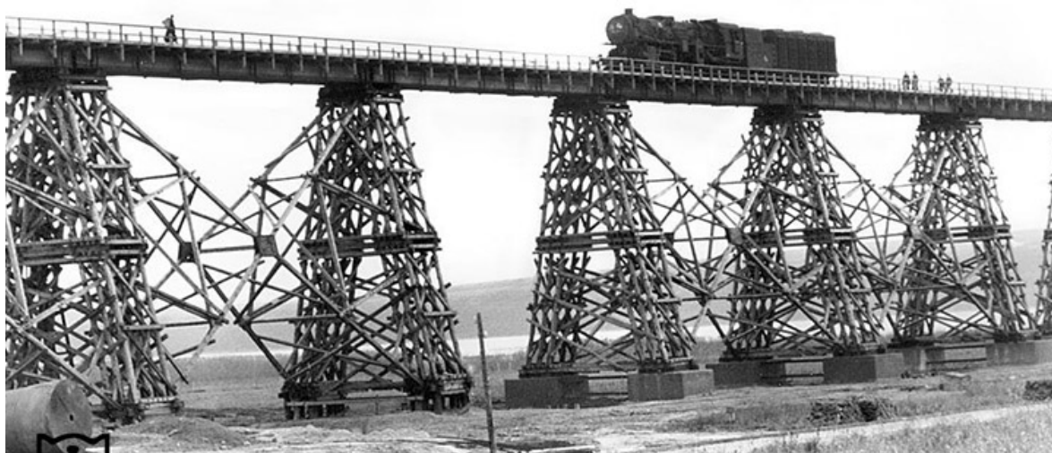
Будівництво трихатського залізничного мосту, 1943 рік
