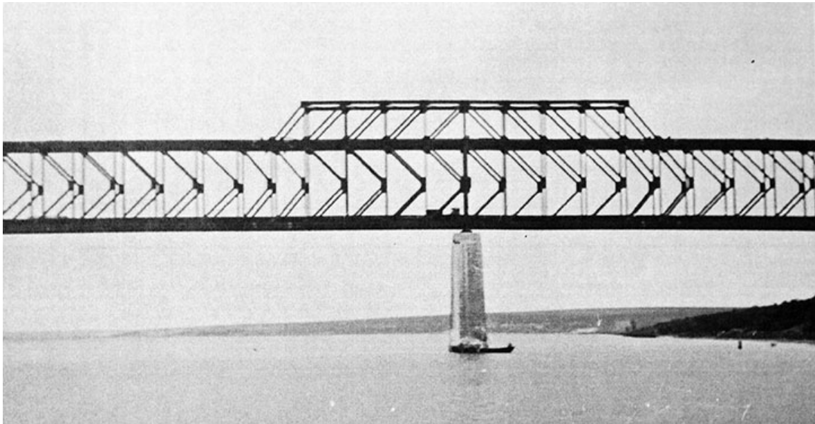
Вид зібраної ділянки мосту з води
