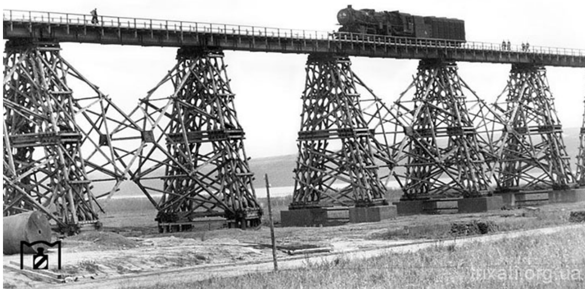
Тестовий проїзд локомотиву BR52 по тимчасовому мосту
